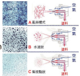
TA-W71A 多功能亂絲噴槍
